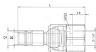
Nippel, drehbar
