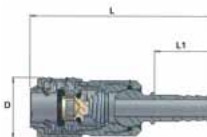
Schlauchtülle, drehbar
