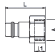
Nippel Innengewinde
