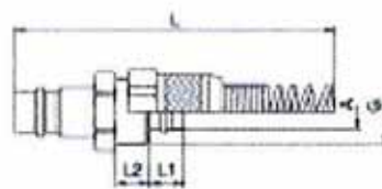
Nippel für Schlauch mit Überwurfmutter und Knickschutzfeder
