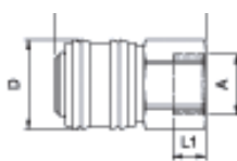
Innengewinde
