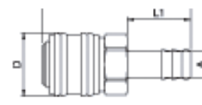
Schlauchtülle
