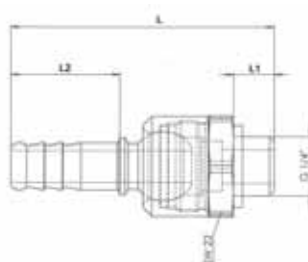
Schlauchtülle, Außengewinde
